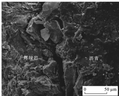
(a) 辉绿岩-沥青
