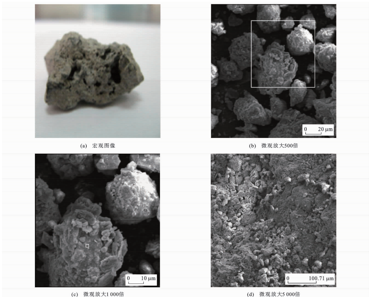
图 1 转炉钢渣形貌特征
