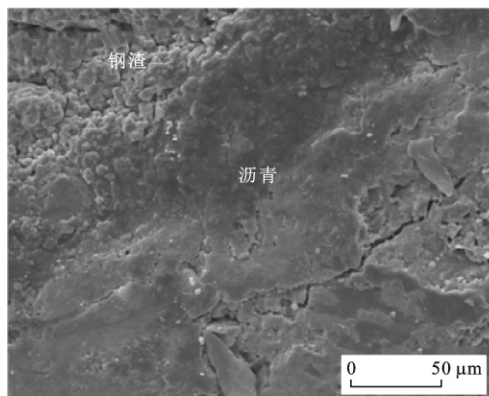
(b) 钢渣-沥青
