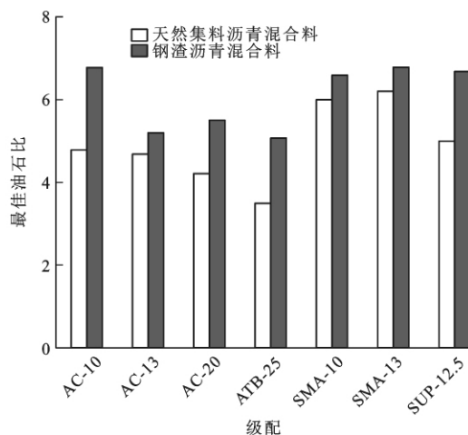
图 6 最佳油石比
