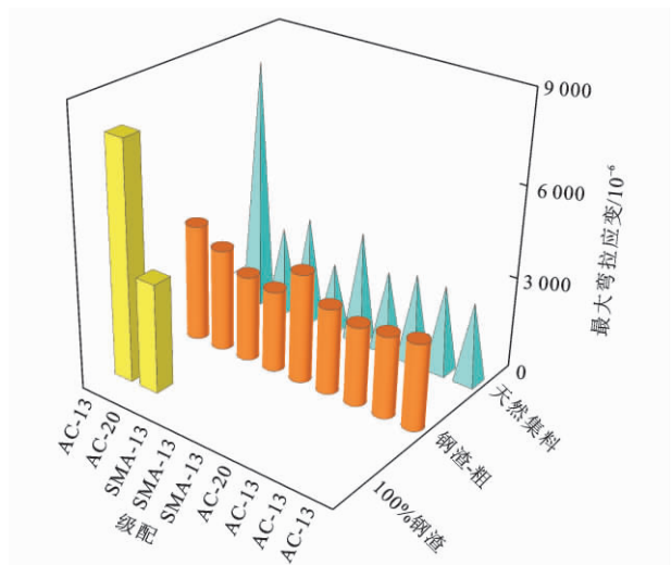
图 8 沥青混合料低温抗裂性
