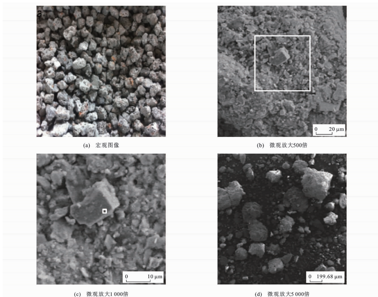
图2 电炉钢渣形貌特征
